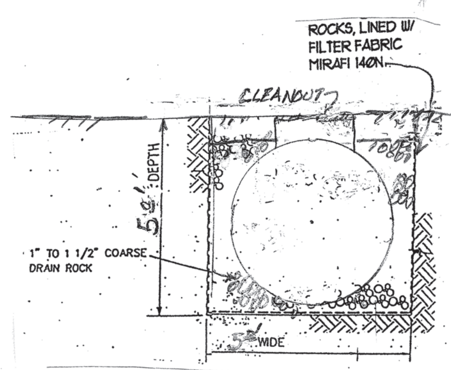
TRENCH SECTION DETAIL (N.T.S.)
